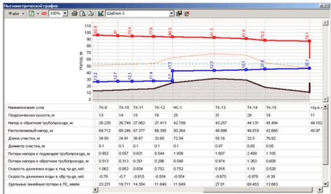
Рисунок 3.13 - Пьезометрический график
