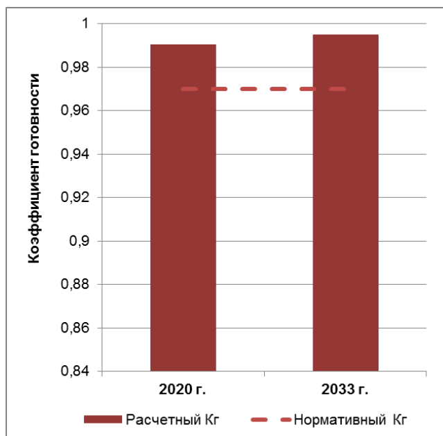
Рисунок 2.2 – Сравнительная оценка средних значений коэффициентов готовности потребителей города Благовещенск
