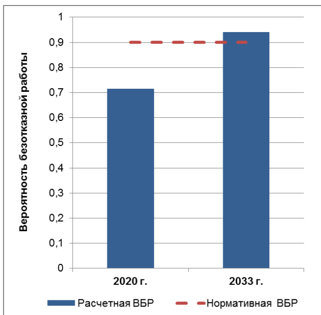
Рисунок 2.1 – Сравнительная оценка средних значений вероятностей безотказной работы потребителей города Благовещенск
