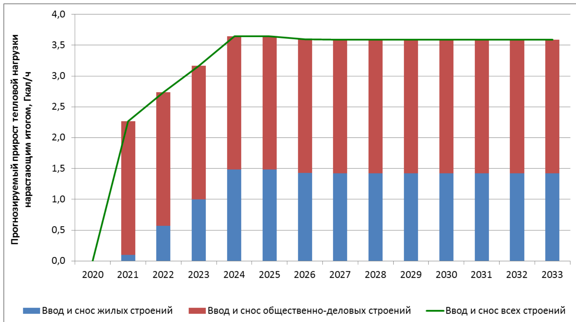
Рисунок 4.2 – Прогнозируемый прирост тепловой нагрузки на территории городского поселения город Благовещенск Республики Башкортостан на период до 2033 года нарастающим итогом (с выделением типов вводимой застройки и сносимых зданий)
