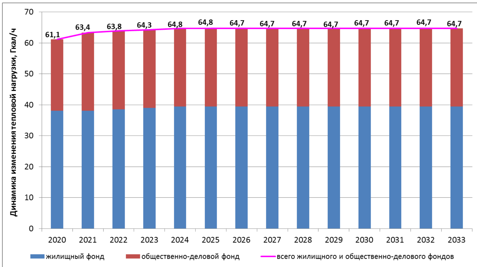
Рисунок 4.4 – Тепловая нагрузка потребителей городского поселения город Благовещенск Республики Башкортостан на период до 2033 года (с выделением типов зданий)
